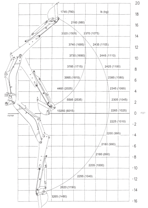
BRAZO TELESCÓPICO, EXTENDIDO
