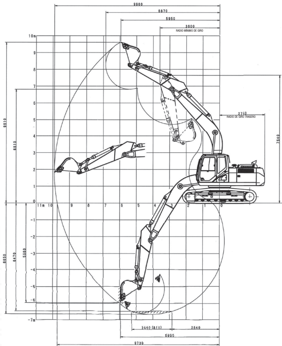
ALCANCE DE EXCAVACIÓN CON BRAZO DE 2,94 M
